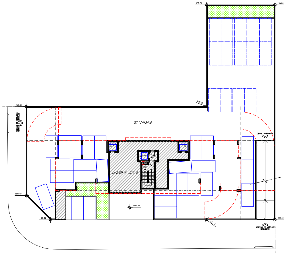
PLANTA TÉRREO
